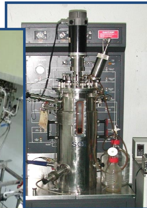
22 L Fermentor
