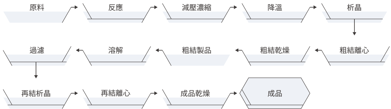
合成流程圖
